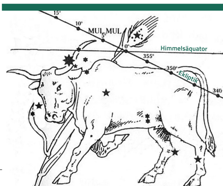
Abbildung 3: Für die Sumerer begann das Jahr, wenn sich die Neulichtsichel des Mondes im Sternbild Stier bei den Plejaden zeigte.
