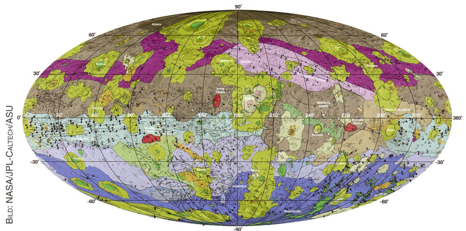
Abbildung 1: Kartierte Vesta.
