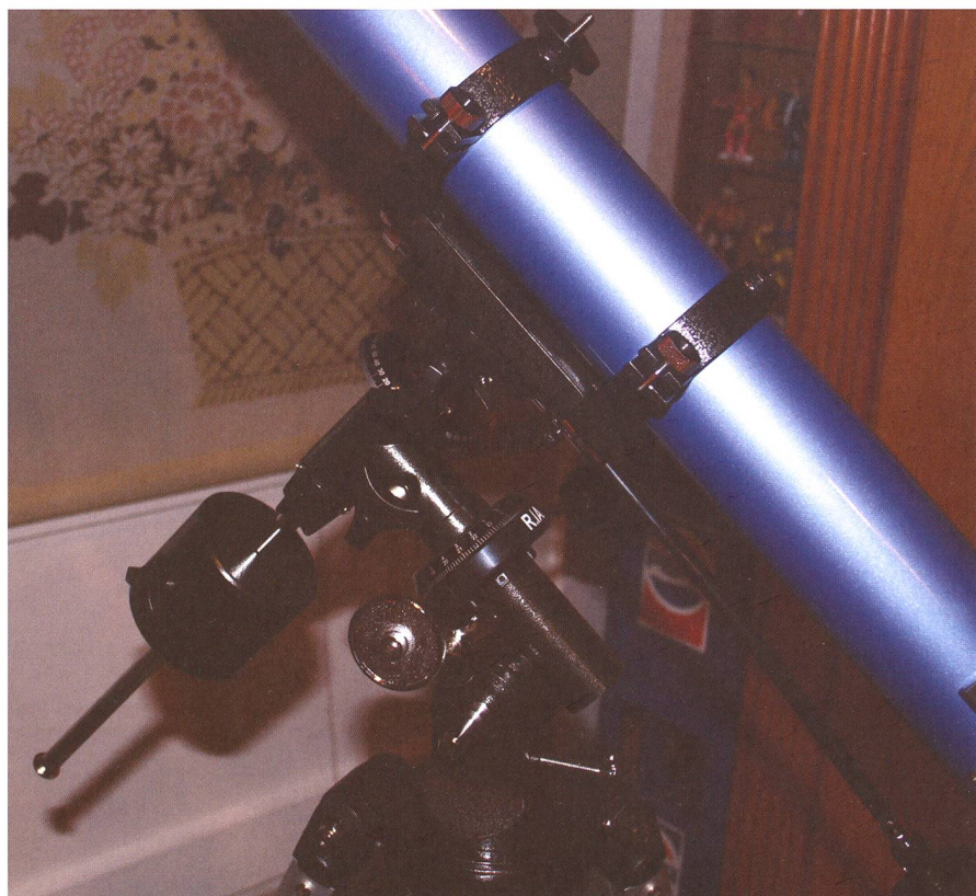
Die EQ-2-Montierung, die mit dem angesetzten 70/900mm-Tubus eine eben noch akzeptable visuelle Stabilität bietet. (Bild: Christian Leu)
