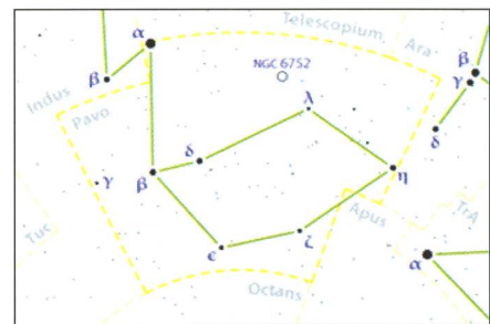
Fig. 2. La constellation du Paon. (© Wikipedia)
