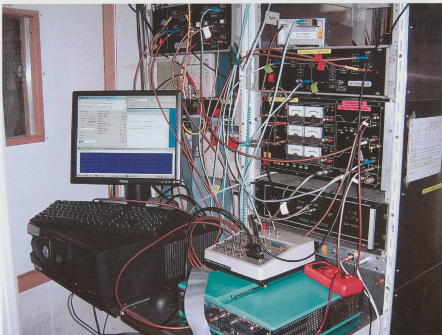
Fig. 1: ARGOS (grüne Kiste rechts unten) im Spektrometerraum des KOSMA auf dem Gornergrat bei Zermatt. Im Hintergrund die Aufbereitung der Zwischenfrequenzen und ein traditionelles AOS. Der PC links vorne steuert das Spektrometer, erledigt die Kommunikation mit dem Teleskop und beherbergt einen FTP-Server für die laufend anfallenden Spektrometer-Daten.
