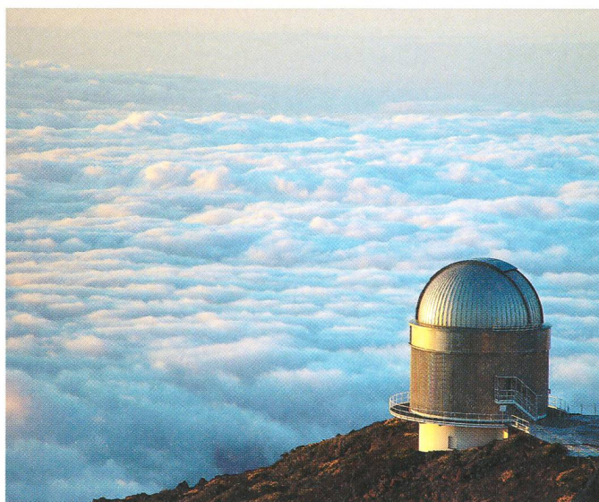
12. Le télescope «Nordic» de 2.5 m installé par un consortium de pays européens nordiques. Cet instrument occupe le site le plus élevé de l'Observatoire et jouit de conditions idéales pour l'imagerie.
