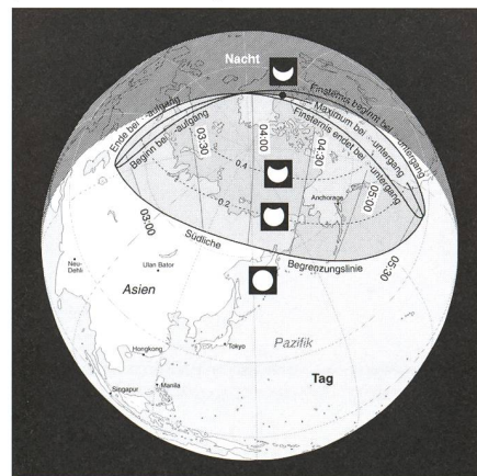
Fig. 2: Partielle Sonnenfinsternis am 31. Juli 2000 auf der nördlichen Erd-Hemisphäre. (Grafik: THOMAS BAER)
