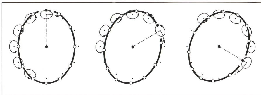
Fig. 2. Cette image montre la trajectoire de forme elliptique imprimée à une étoile dans son mouvement autour du centre de la galaxie par l'ensemble des forces gravitationnelles à longue distance qu'elle subit. La trajectoire réelle de l'étoile est une succession d'épicycles centrés sur l'orbite elliptique, produit par les perturbations gravitationnelles des objets de son environnement immédiat.
