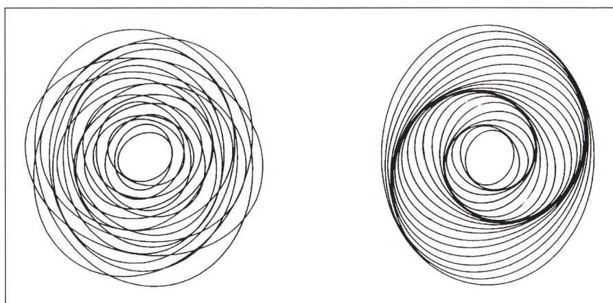
Fig. 3. Les deux dessins contiennent exactement le même nombre d'ellipses. Dans celui de gauche l'orientation des grands axes est aléatoire; par contre, dans celui de droite, chaque grand axe est légèrement pivoté par rapport au précédent. La zone des bras spiraux apparaît très clairement.
