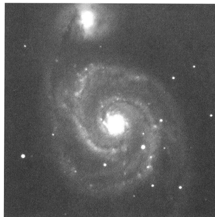
Spiralnebel M 51 in den Jagdhunden. Galaxie M 51 dans les Chiens de Chasse. Aufnahme vom/Cliché du 11.4.97, 1:04 UT ( \alpha = 13^h 29^m 54^s , \delta = +47^\circ 12' ), B-Filter: 600 s, V-Filter: 200 sec, R-Filter: 120 s, I-Filter: 120 sec.
