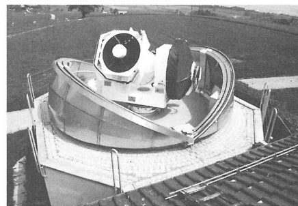
ZIMLAT auf seiner azimutalen Gabelmontierung. In seiner Öffnung der Sekundärspiegel und rechts, am Ende der Horizontalachse, die Plattform mit den Kameras (schwarze Trommel). ZIMLAT sur sa monture à fourche azimutale. Dans son ouverture le miroir secondaire et à droite (tambour noir) la plate-forme portant les caméras.
