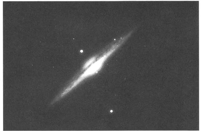
NGC 4565
