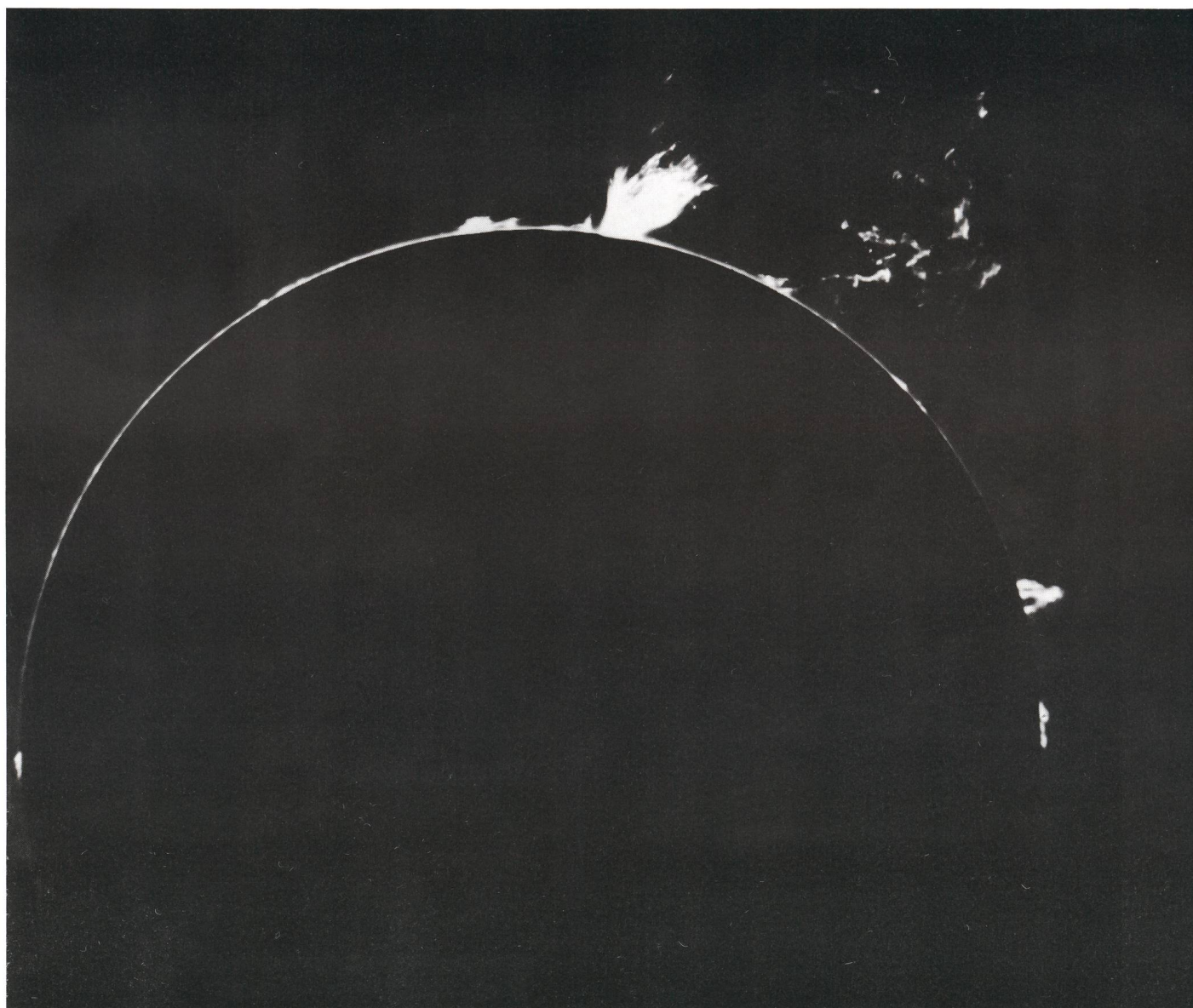
Protuberanzausbruch am Sonnenrand vom 26. März 1989, 14.20 Uhr WZ. Höhe: 400 000 km, Länge: 600 000 km. Sonnenteleskop 90/1 300 mm und 9 Å H - Alpha - Filter, TP 2415, 1/60 Sek. Aufgenommen in Puimichel/Haute Provence (Frankreich). GERHARD KLAUS, Waldegstrasse 10, CH - 2540 Grenchen.
