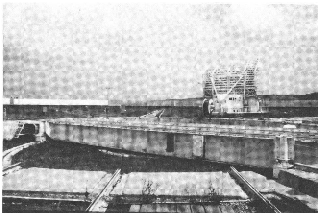
Ausschnitt der im Durchmesser 600 m messenden Anlage.
