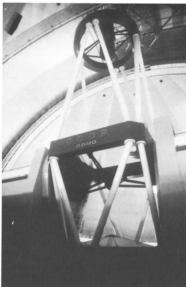
Ansicht des Riesenteleskopes (Höhe 42 m, Durchmesser 6 m, Gewicht 1 200 Tonnen).
