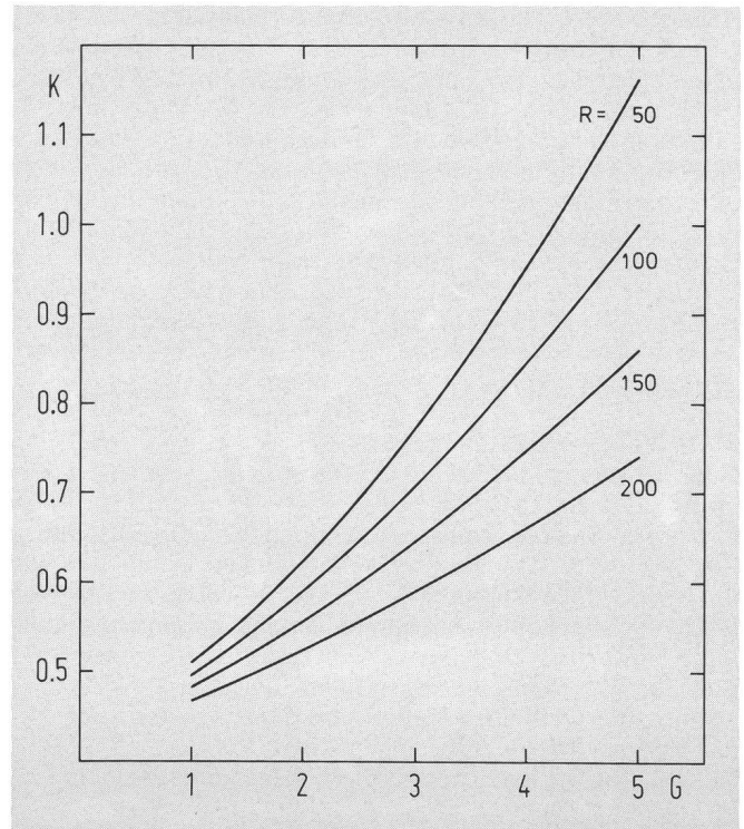
Abb. 5: Abhängigkeit des k-Faktors von der Luftgüte G (Mittel aus Luftruhe und Bildschärfe) nach 10) aufgetragen für verschiedene Werte der Relativzahl R , normiert auf k = 1.0 bei G = 5 und R = 100 .
