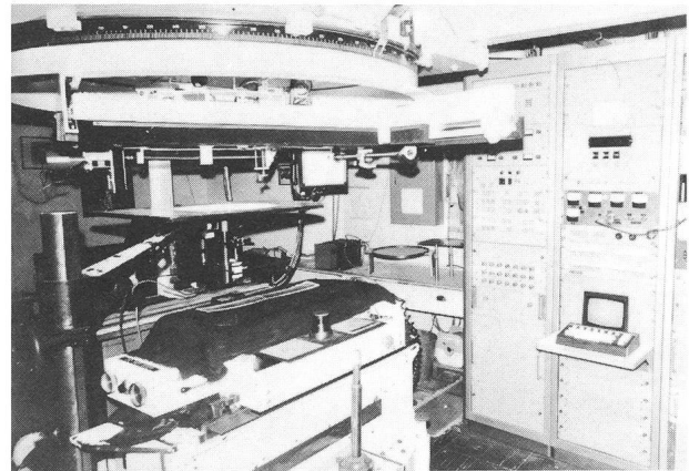
Abb. 3: Das Innere des 50-m-Sonnenturms. Heute werden hier hauptsächlich die Magnetfelder der Sonne vermessen. Das Sonnenbild erscheint auf der von links einschwengbaren Platte in einem Durchmesser von etwa 40 cm. Aufnahme: M. Lammerer
