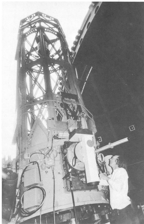
Abb. 5: Der 60-Zöller auf dem Mt. Wilson. Bei seiner Inbetriebnahme 1908 war dieses Instrument das grösste Fernrohr der Welt. Heute ist es mit moderner Elektronik ausgestattet wie dem Photonen-Zähler, der hier im Cassegrain-Fokus des Instruments Anwendung findet.
