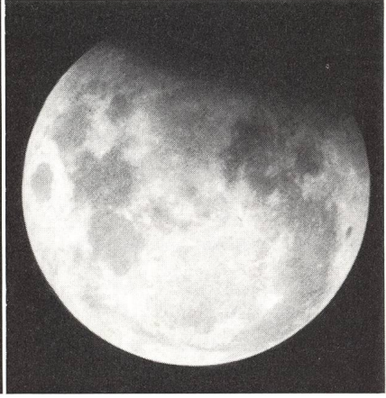
Bild 3 Aufgenommen 10. 12. 73 02.44 Uhr MEZ Belichtungszeit 1 s Maximum der Finsternis
