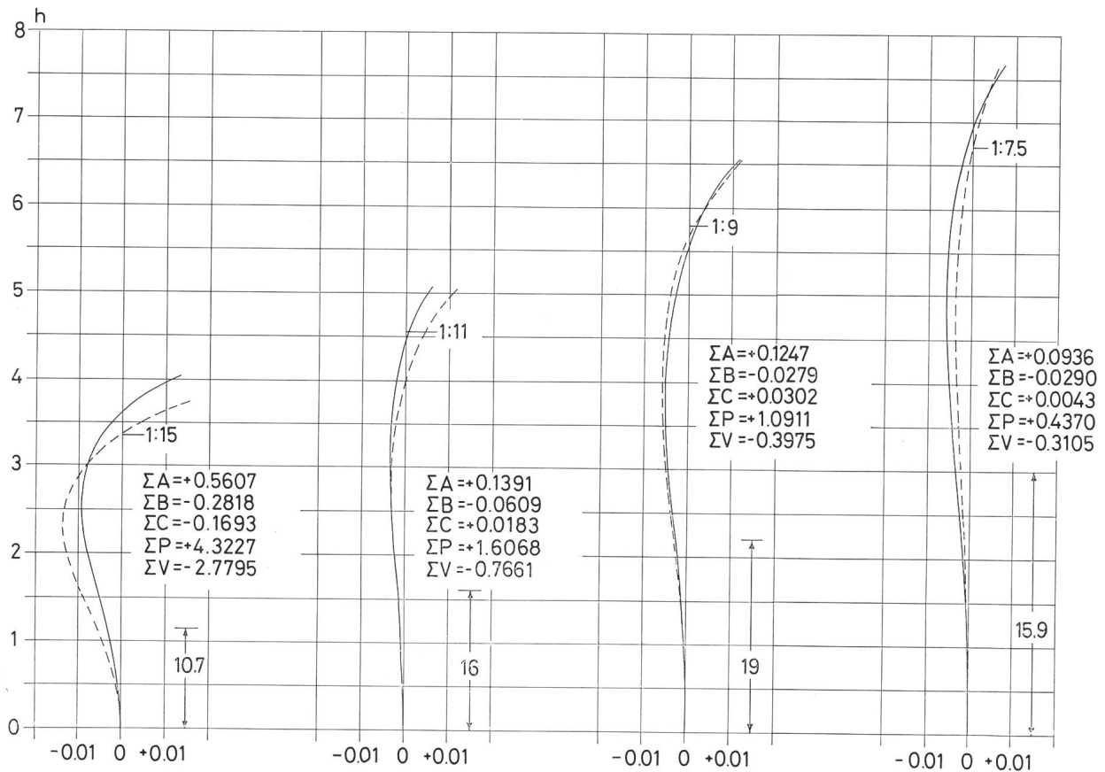
Fig. 2: Systemschnitte mit den Öffnungen: 1:15, 1:9 und 1:7,5.
