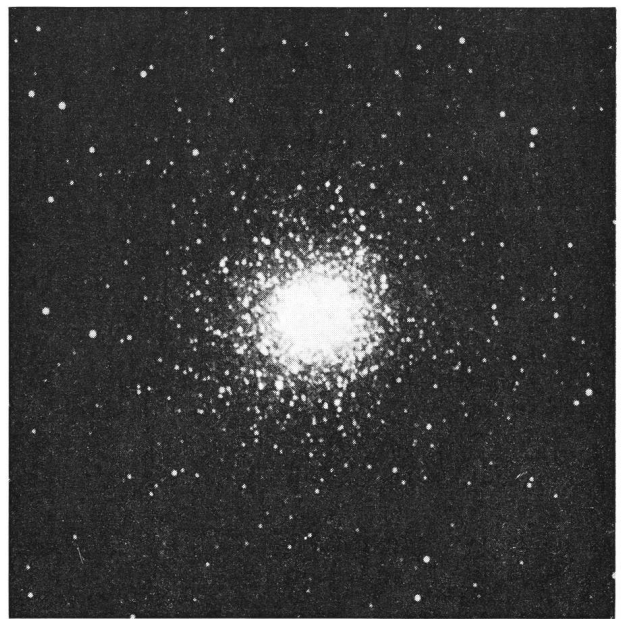
Kugelhäufen M 13, Belichtungszeit 50 min auf Tri X Pan.
