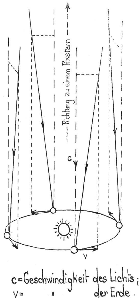
Fig. 3 Aberration des Lichts
