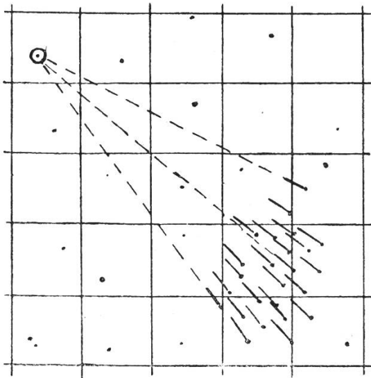
Fig. 5 Konvergenzpunkt der Eigenbewegungen in einem offenen Sternhaufen
