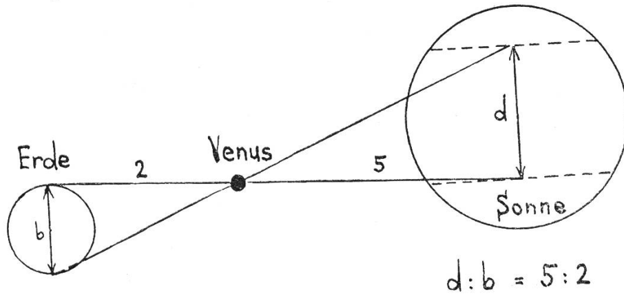
Fig. 2 Venusdurchgang
