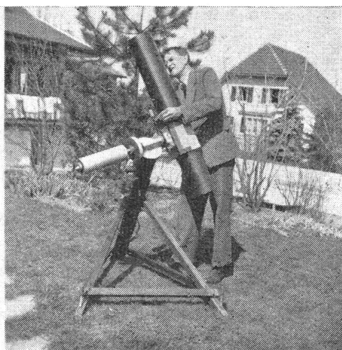
Bedienung der Feinbewegungen
