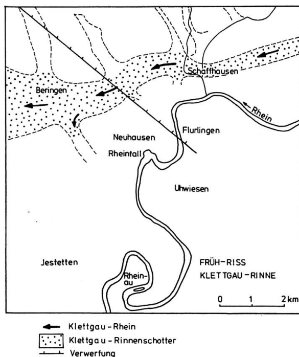
Fig. 6 In der Zwischeneiszeit zwischen Mindel- und Rissvergletscherung floss der Rhein von Schaffhausen durch den Klettgau nach Westen.
