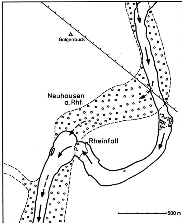
Schotter der zwischeneiszeitlichen Rheinrinne — zwischenzeitlicher Rheinlauf — heutiger Rheinlauf — Verfurgung
