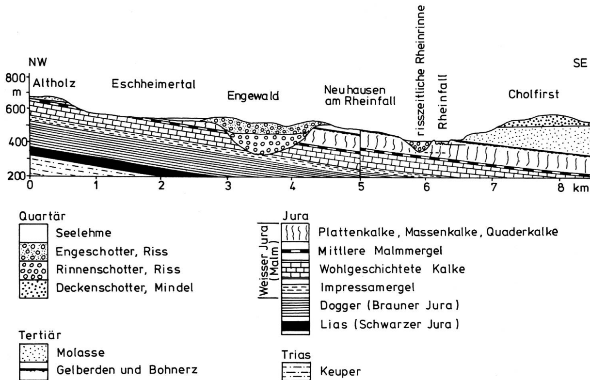
Fig. 3 Geologisches Querprofil durch das Rheinflallgebiet vom Randen zum Cholfirst. In der Umgebung des Rheinfalls treten von der Juraformation nur die höchsten Kalksteinlagen zu tage. Das Profil zeigt, welche Schichten in der Tiefe zu erwarten sind. Eine am Rheinfall angesetzte Tiefbohrung würde unter den Jura- und Triasschichten in etwa 700 m Tiefe auf das sogenannte Grundgebirge stossen, wie es im Schwarzwald zum Vorschein kommt (vermutlich Gneis oder Granit).
