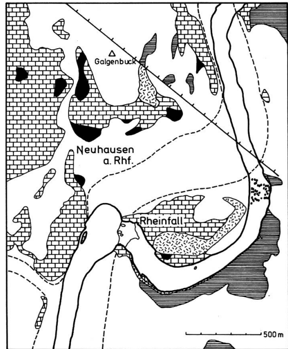
eiszeitliche und jüngere Ablagerungen Molasse Gelberden (Altligozän) — Verfurgung Bohnerz (Eozän) Kalksteine des oberen Weissen Jura (Malm)
