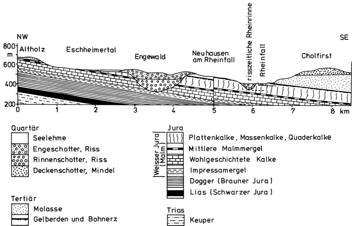
Fig. 3 Geologisches Querprofil durch das Rheinflalgebiet vom Randen zum Cholfirst. In der Umgebung des Rheinfalls treten von der Juraformation nur die höchsten Kalksteinlagen zutage. Das Profil zeigt, welche Schichten in der Tiefe zu erwarten sind. Eine am Rheinfall angesetzte Tiefbohrung würde unter den Jura- und Triasschichten in etwa 700 m Tiefe auf das sogenannte Grundgebirge stossen, wie es im Schwarzwald zum Vorschein kommt (vermutlich Gneis oder Granit).
