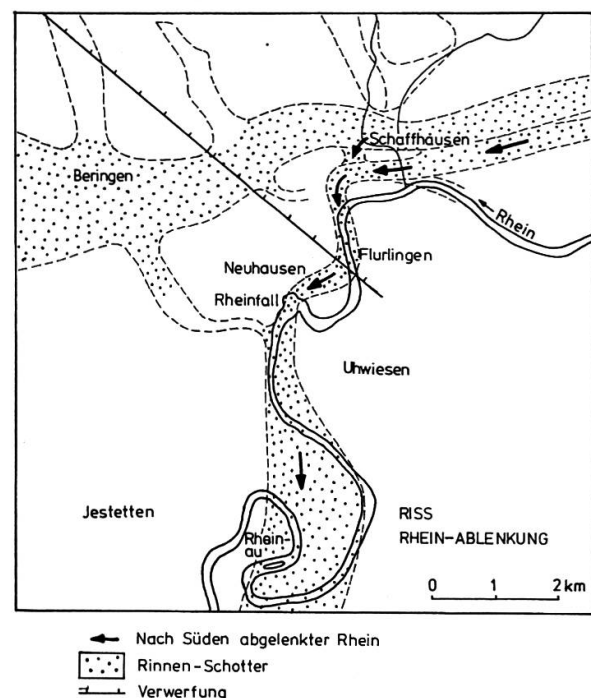
Fig. 7 Während der Risseiszeit wurde der Rhein von Schaffhausen nach Süden abgelenkt. Der Klettgau wurde trockengelegt, nachdem sein Tal mit Schottern aufgefüllt worden war.
