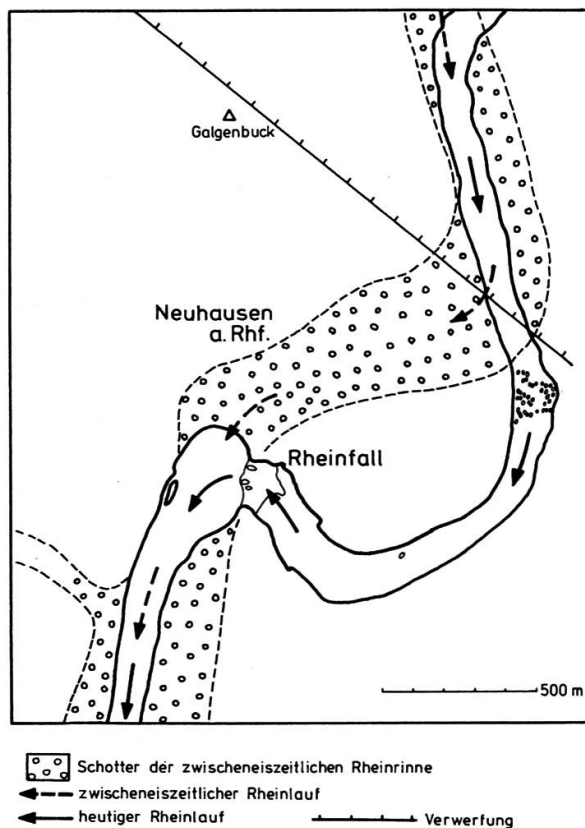
Fig. 8 Verlauf der risseiszeitlich entstandenen Schotterrinne des ehemaligen Rheinlaufs, die Anlass zur Entstehung des Rheinfalls gab: der Rhein stürzt von Osten her über die Felswand der ehemaligen Schlucht in sein altes Tal, aus dem er vom Rheinfallbecken an flussabwärts die Schotter ausräumte.
