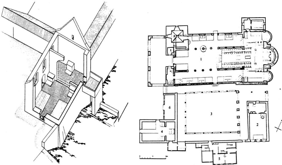
Rekonstruktion der barocken Galluskapelle von 1638 bis 1642, Nr. 4 auf dem Grundriss des engeren Stiftsbezirks (Aus "Das Stift Beromünster")
