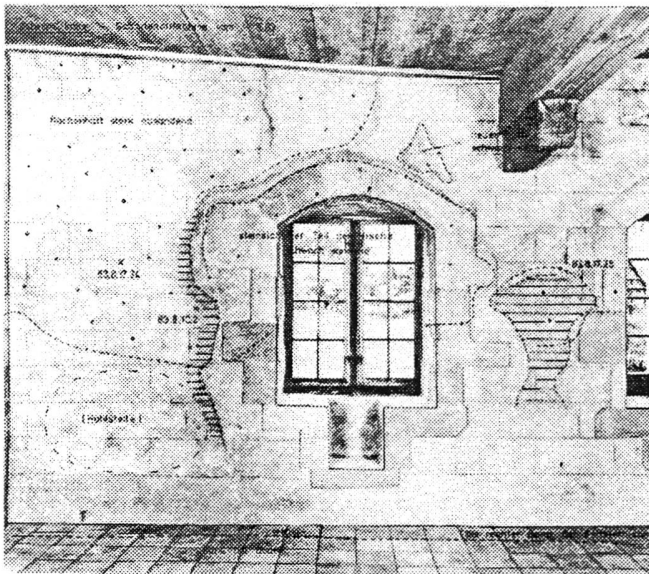
Schadensaufnahme im ehem. Kloster in Kappel a.A. (Aus "Zürcher Denkmalpflege, 10. Bericht, 1. Teil")
