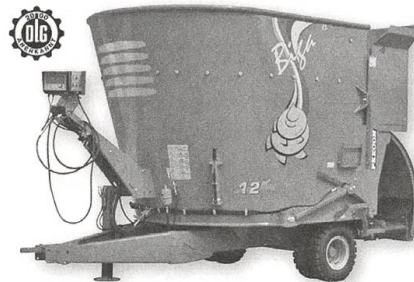
Futtermischwagen PEECON mit Verlade-Einrichtung
