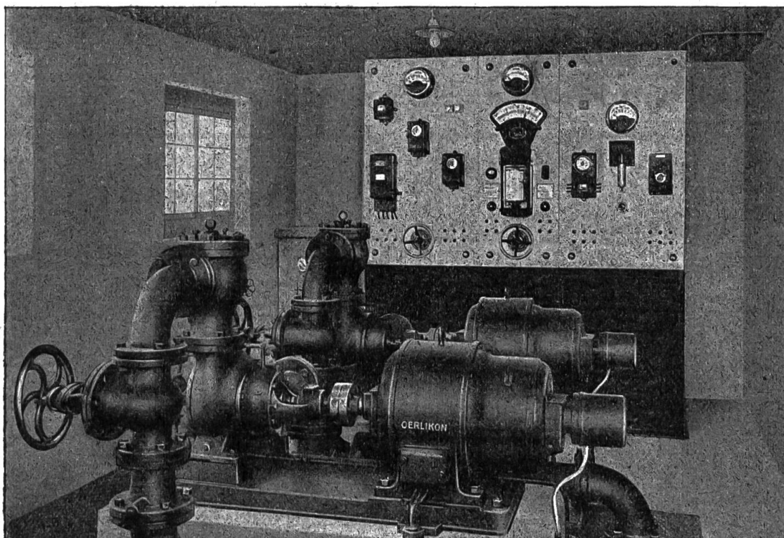
Automatische Pumpen-Anlage einer Wasserversorgung.
