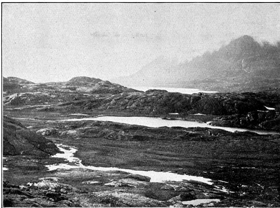
Fig. 1. See No. 1. von Holstensborg. (Im Hintergrund das Meer.) Rundhöckerlandschaft. 21. VI. 1908.
