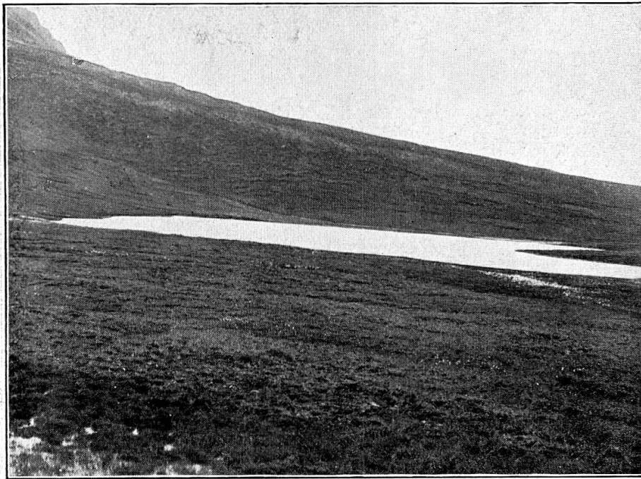
Fig. 5. Teich No. 76 am Skarvefield. 15. VIII. 1908.
