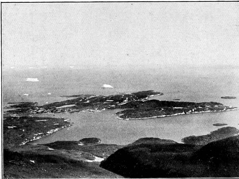
Fig. 8. Übersicht von Godhavn. Fläche vom Gletscher gehobelte Halbinsel d. Insel Disko. Links d. See No. 29. Rechts See No. 61. (20. VII. 1908.)
