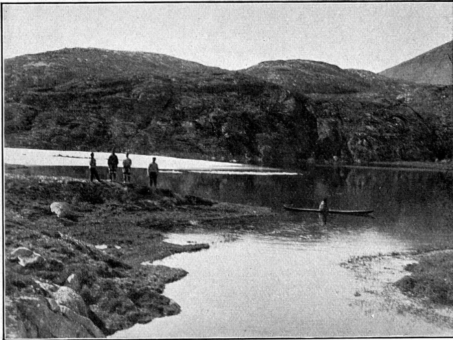
Fig. 7. See No. 72 des Diskofiord. 13. VII. 1908.
