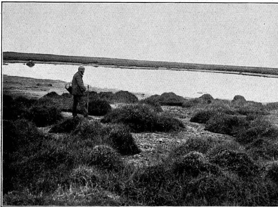
Fig. 4. Verlandeter flacher See auf Nordfiord. Im Vordergrund „Maulwurfhügellandschaft“ 7. VIII. 1908.
