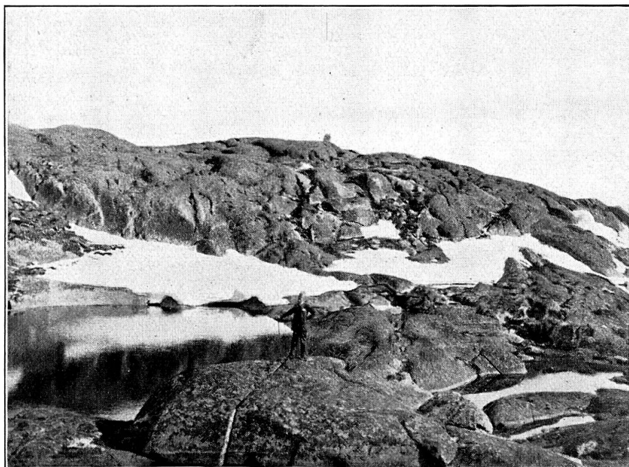
Fig. 2. Gneisteich No. 4 von Godthaab. Typisches Felsbecken in Rundhöckerlandschaft. 14. VI. 1908.
