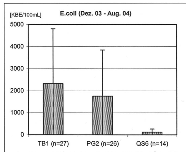
Abb. 10: Darstellung aller bisherigen Messungen bezüglich der Veränderung der Fäkalkeimzahl ( E. coli ) während der Passage durch das Pflanzenklärgbiet und durch den Quellsee (TB1 = Einlauf ins Pflanzenklärgbiet, PG2 = Einlauf in Quellsee, QS6 = Auslauf aus Quellsee). Die Abnahme im Pflanzenklärgbiet beträgt 25%, im Quellsee ist die Zahl gegenüber dem Birswasser um 93% zurückgegangen.
