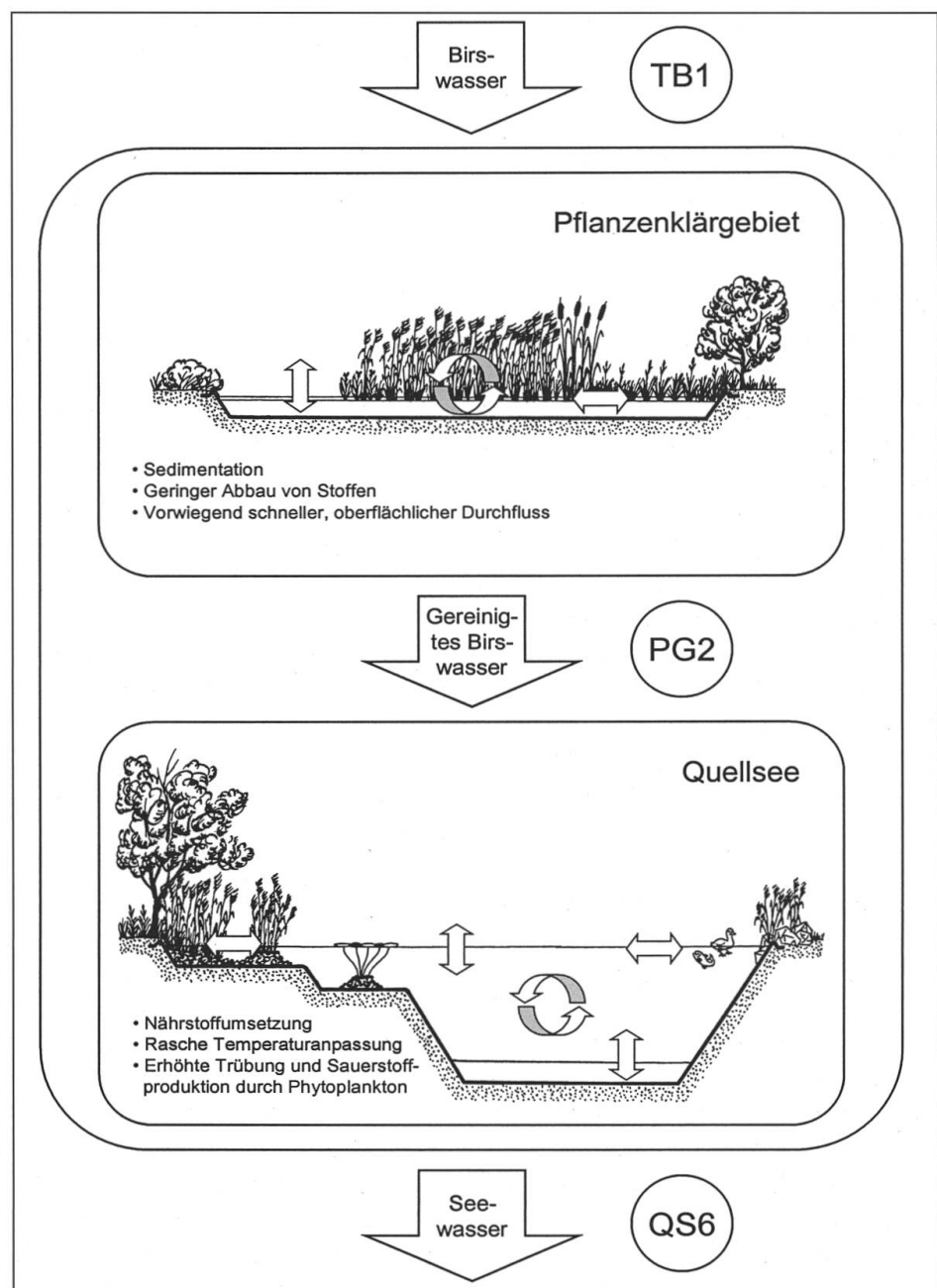
Abb. 3: Das Gewässersystem in der Brüglinger Ebene kann vereinfacht als Black box (Input: Birswasser, Output: Seewasser) oder als Grey box mit den beiden Stufen Pflanzenklärgebiet (Input: Birswasser, Output: gereinigtes Birswasser) und Quellsee (Input: gereinigtes Birswasser, Output: Seewasser) betrachtet werden. Spezifische Untersuchungen im Pflanzenklärgebiet und im Quellsee vertiefen die Erkenntnisse über ablaufende Prozesse in den jeweiligen Reinigungsstufen (Messpunkte: TB1 = Einlauf ins Pflanzenklärgebiet, PG2 = Einlauf in Quellsee, QS6 = Auslauf aus Quellsee).
