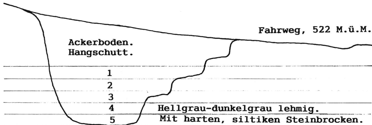
Querschnitt durch den Hang. Graben-Profil. Jura-Nagelfluh* bis auf 581 m über Meer. * Schwarzwald-Geschiebe-Schotter. Miocæn, Tortonien, 10–15 Mio. Jh.
