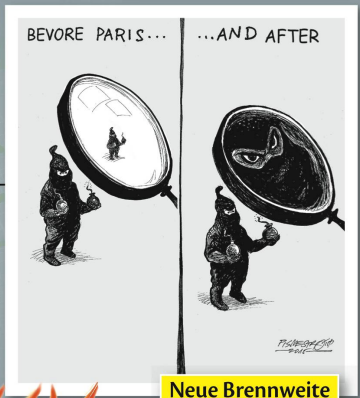
Neue Brennweite
