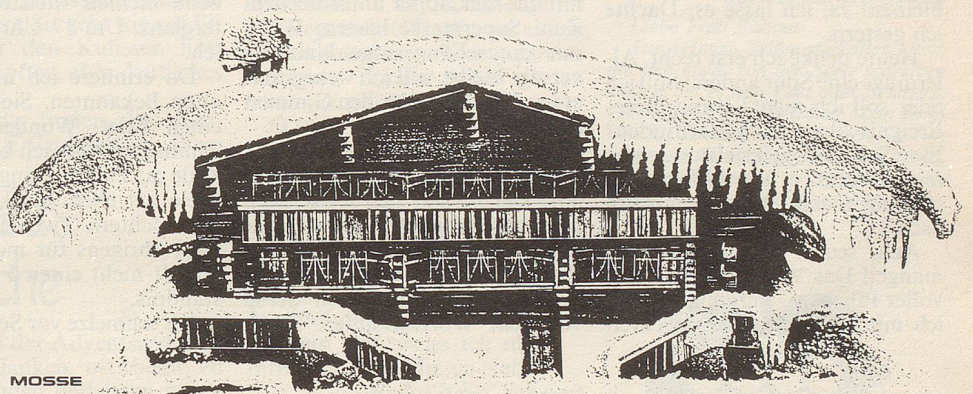
MOSSE
