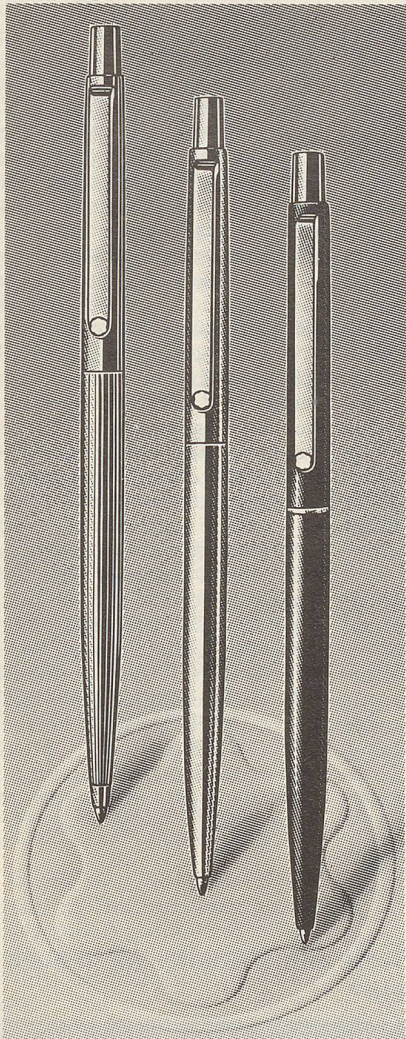
MOSSE
