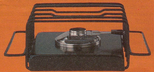
2150-6 Firestar-Rechaud, rechteckige Form 28x20 cm, Rost und Griffe aus rostgeschütztem Schmiedeeisen schwarz, Unterteil aus schwarzem Stahlblech, herausnehmbar, Brenner aus Chromnickelstahl 18/10
