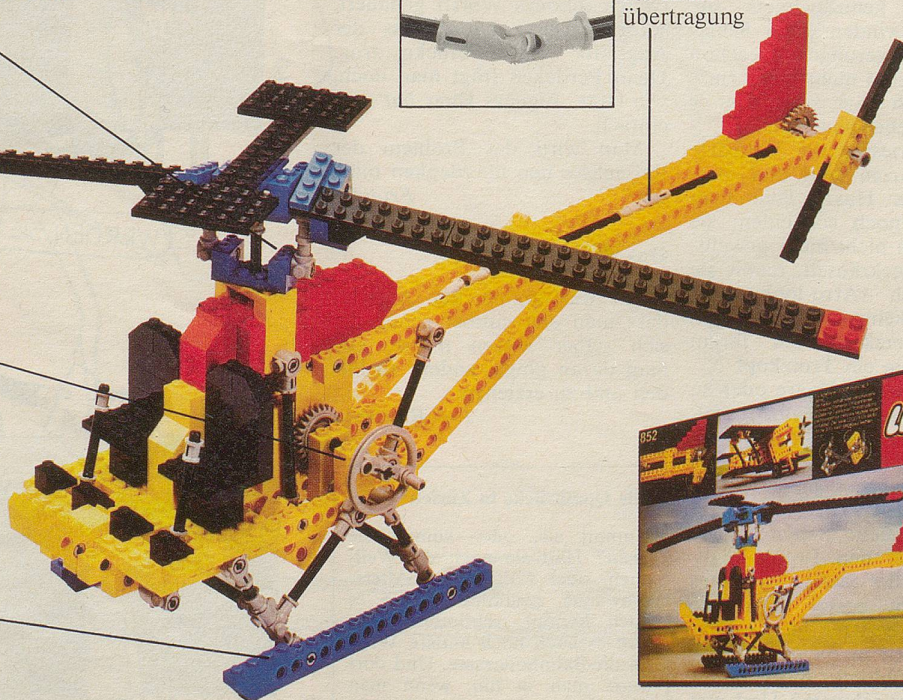
Bewegung durch Lochsteine und Buchsen
