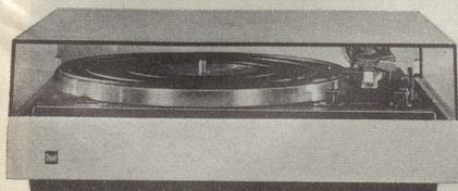
CS 70 Hi-Fi-Stereo-Automatikspieler Dual 701 mit elektronischem Zentralantrieb Dual EDS1000. Gerät der absoluten Spitzenklasse. Tonabnehmersystem Ortofon M 20 E mit elliptischem Abtastdiamant. Komplett mit Sockel und Haube, spielbereit. Nussbaum Fr. 1225.-, Weiss Fr. 1245.-
