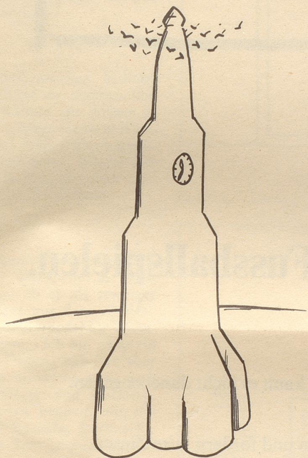
Interplanetarische Zeit
