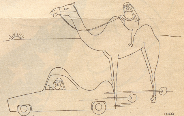
Modell Sahara
