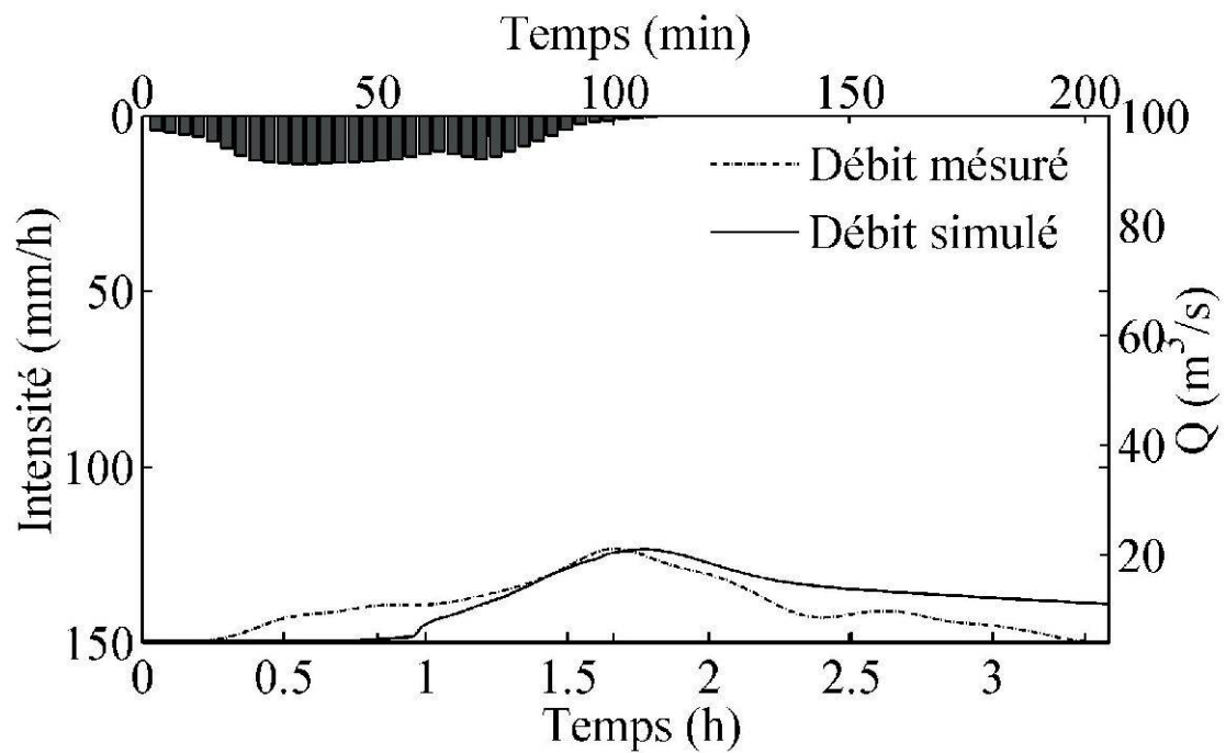
Figure 8.—Hyétoqramme de la pluie et hydrogramme de la crue (24.08.2004). Hyetograph of the rain and flood the hydrograph (24.08.2004).
