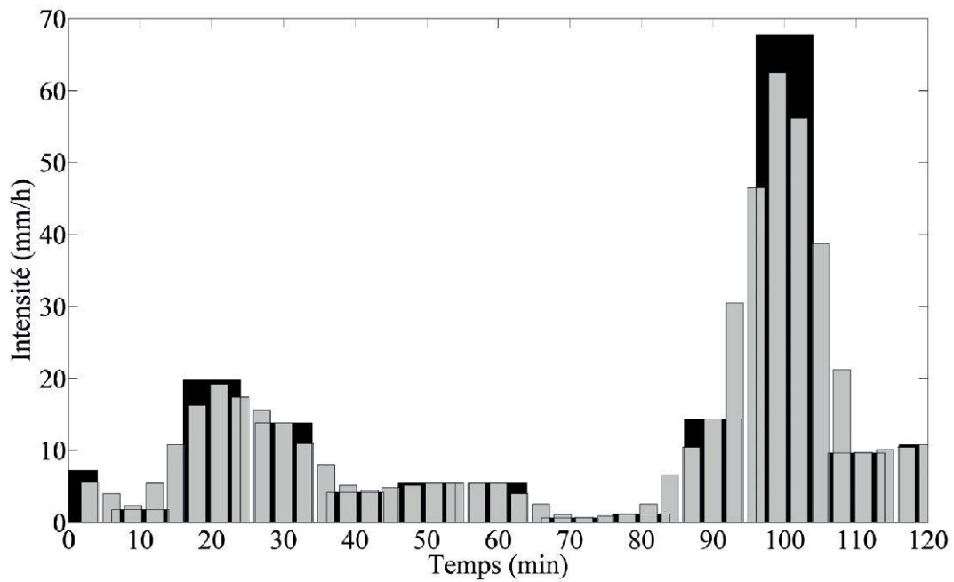
Figure 5.–Hyétogramme de la pluie (07.08.200). Hyetograph of the rain (07.08.2004).
