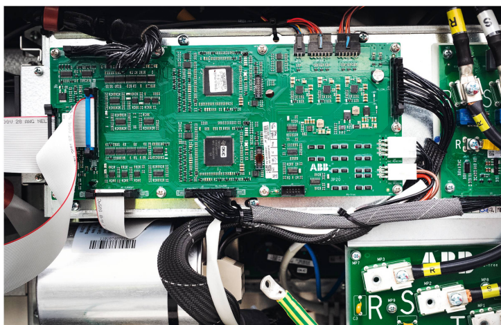
100 kilowatt di potenza: l'interno di un inverter fotovoltaico.
