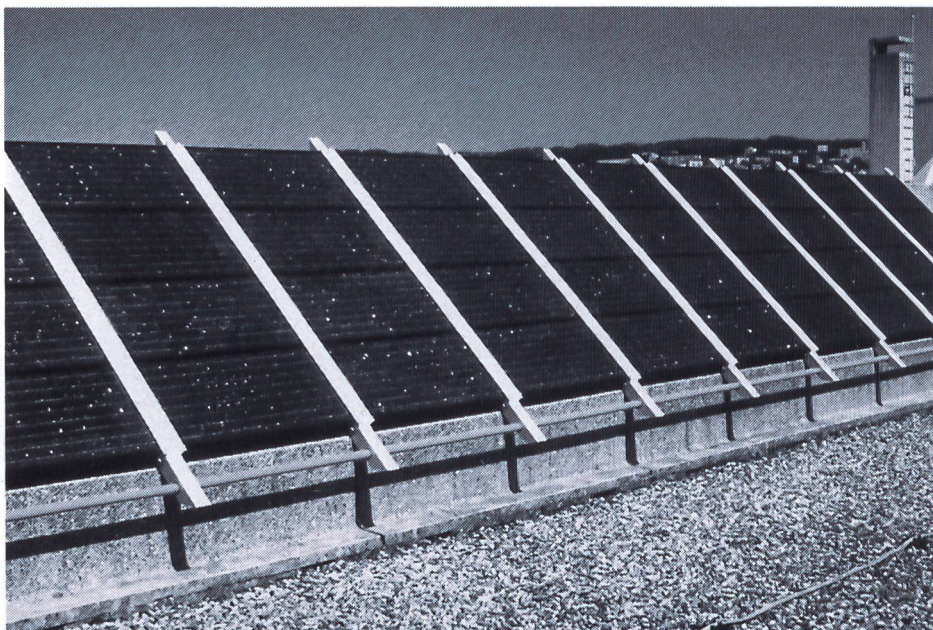
Integrazione architettonica del fotovoltaico: installazione di 3kW collegata alla rete e montata su un tetto della SPFL. (Fotografie LESO/SPFL)
