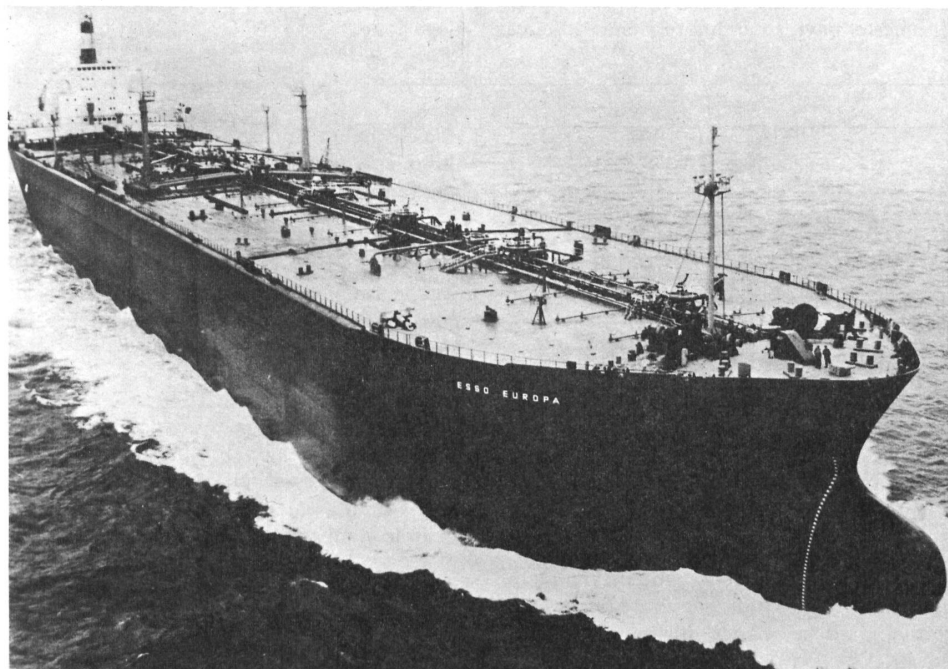
La superpetroliera Esso Europa, lunga 348 m. e larga 52 m., con una capacità di carico di 250.000 dwt. (1 deadweightton = 1016 kg.) Per ragioni di stabilità, l'immensa cisterna che costituisce lo scafo di una petroliera è divisa in compartimenti, con parecchie decine di serbatoi. Questa suddivisione offre il vantaggio di poter caricare, durante lo stesso viaggio, prodotti diversi. Se il petrolio viene raffinato — almeno in parte — nello stesso paese d'origine, le petroliere possono così trasportare non solamente il greggio ma anche benzina, gasolio, olio combustibile, ecc.
