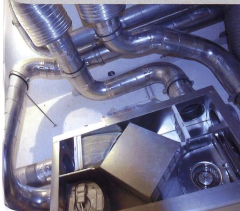
Point névralgique de la ventilation, l'aspiration d'air frais dans la chaufferie.
