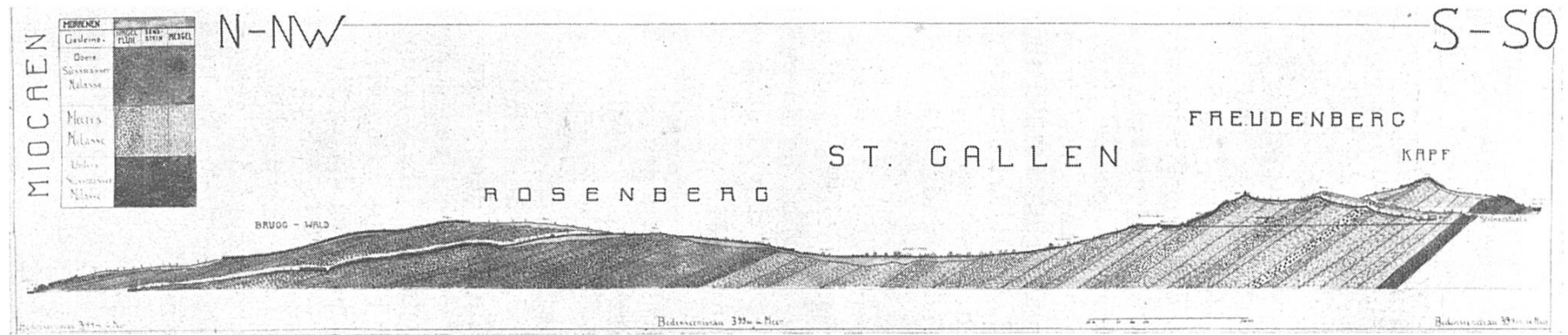
29. Geologisches Profil Rosenberg-Freudenberg nach Dr. G. Rüetschi.
