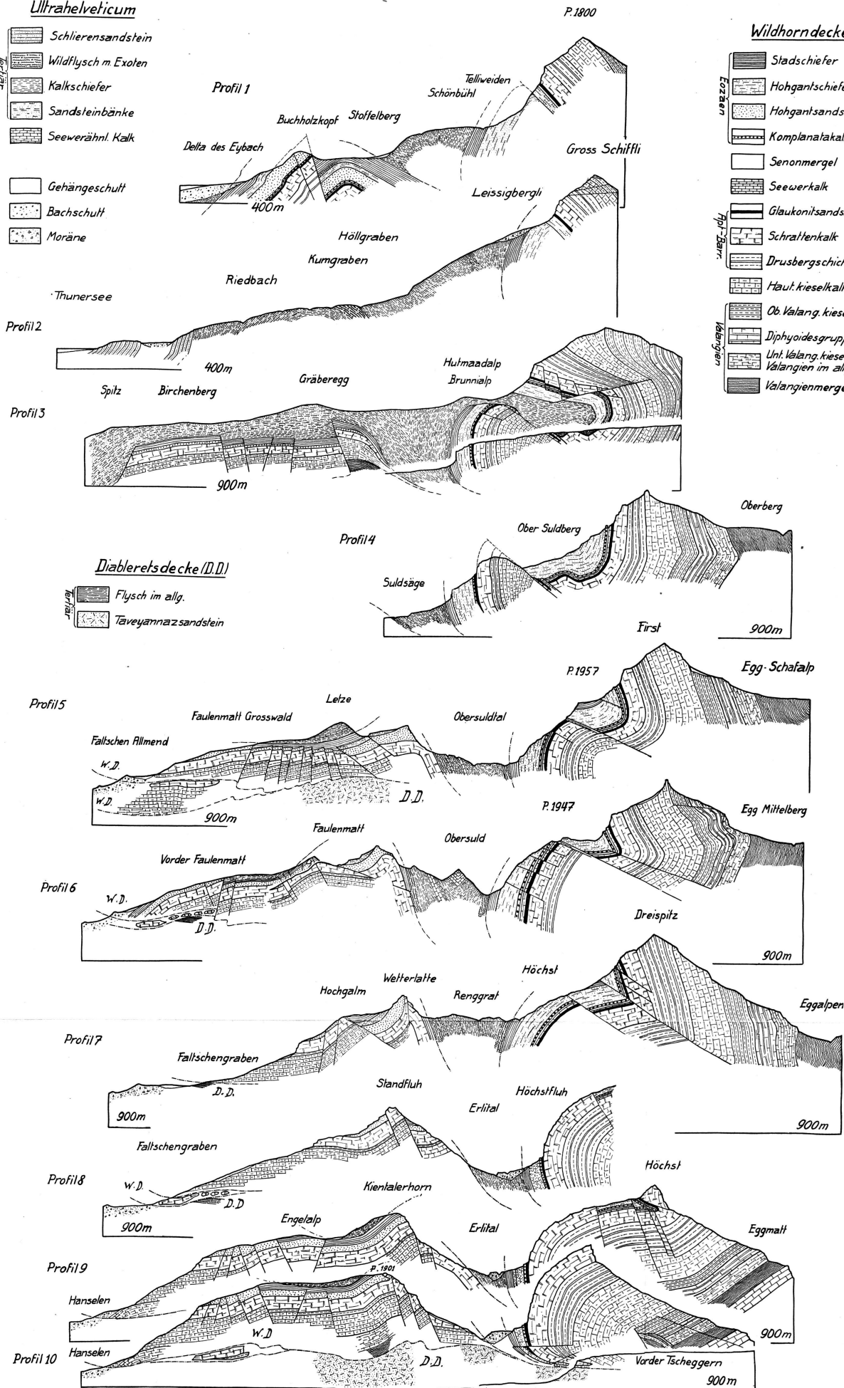
Querprofile durch die Dreispitz-Standfluhgruppe und die Flyschregion südlich des Thunersees
