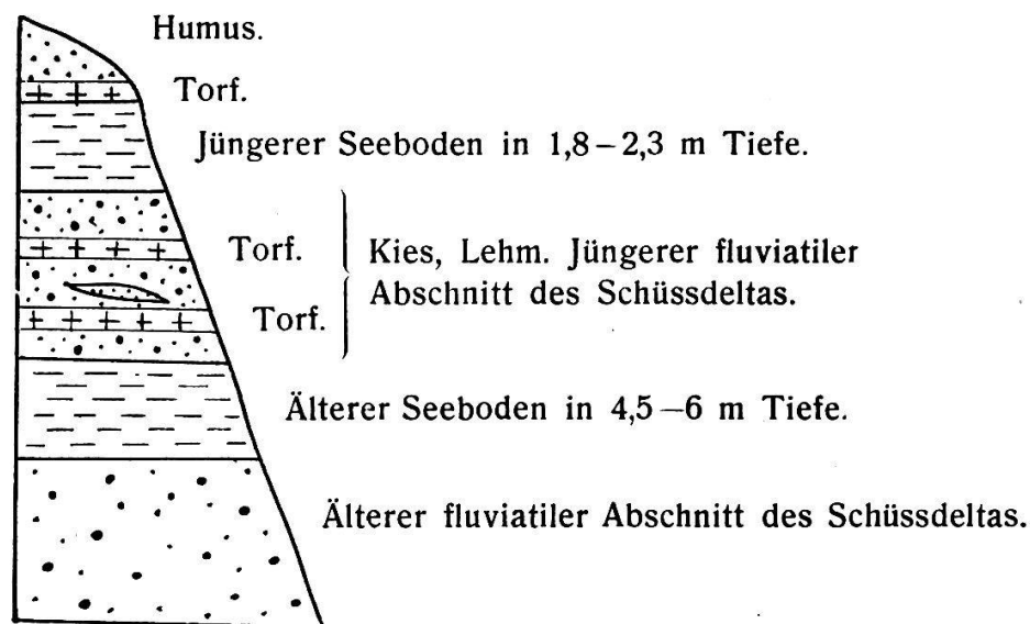
Abbildung 2. Schuttkegel der Schüss bei Nidau.
