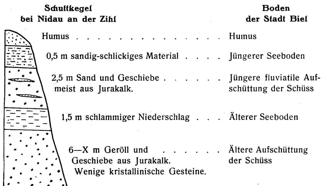
Abbildung 1. Der Alluvialboden der Stadt Biel.
