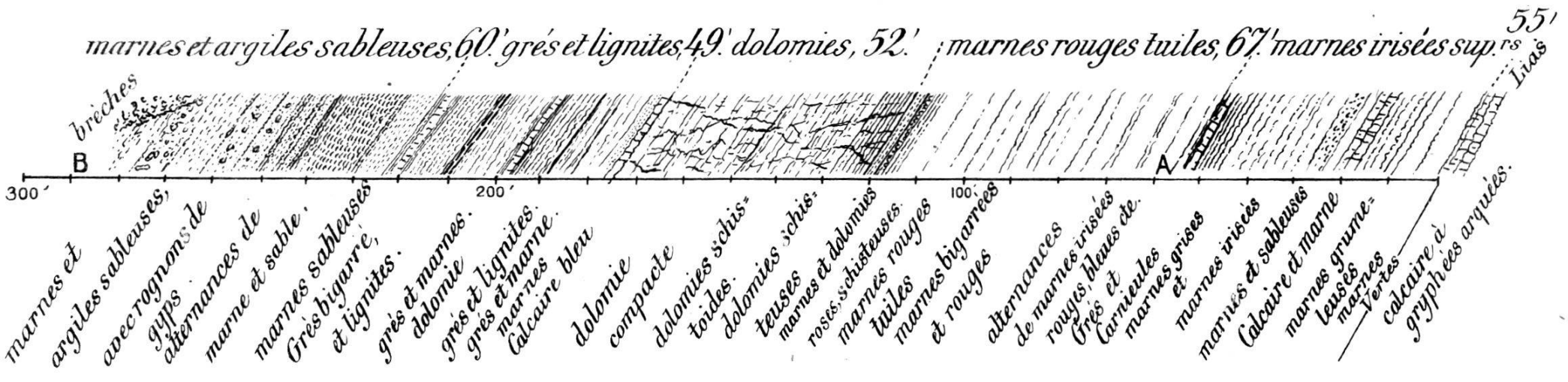
Coupe géométrique des terrains soulevés au Vorbourg et à Bellerive .
