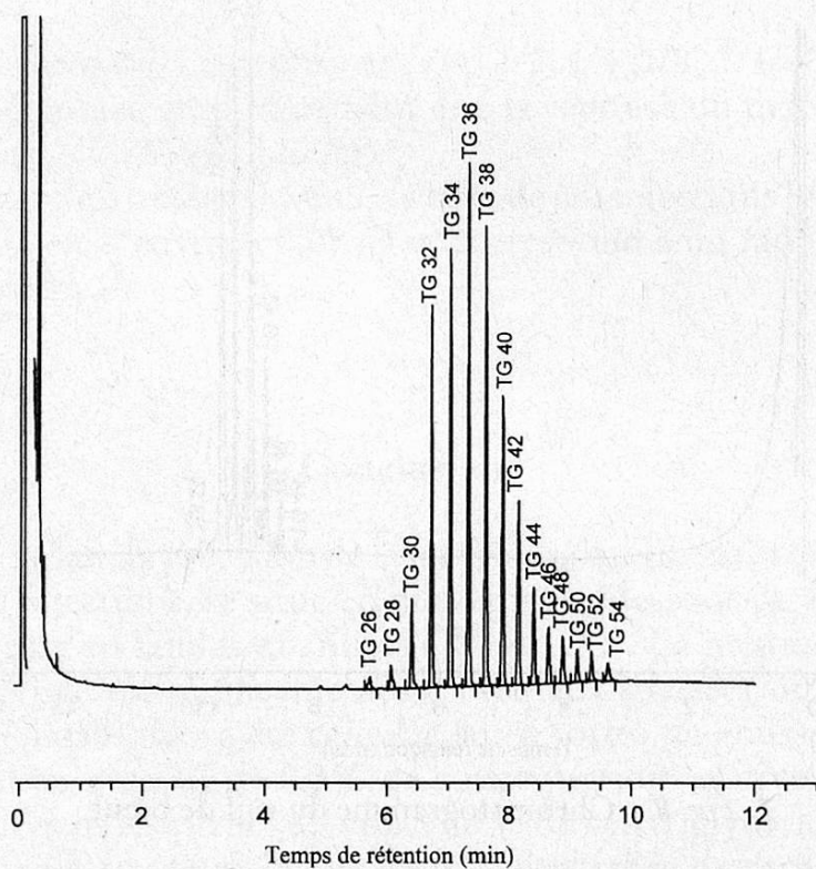
Fig. 6. Chromatogramme de la graisse de coprah
