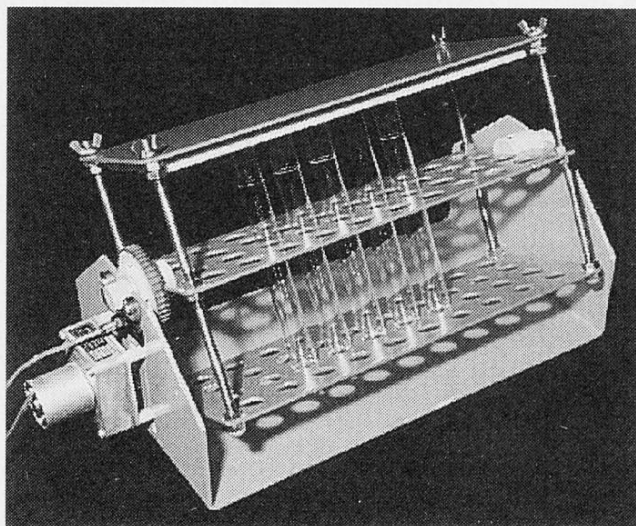
Abb. 1. Rotationsmischer
