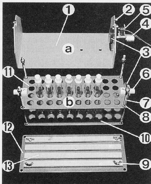
Abb. 2. Details zu Rotationsmischer
