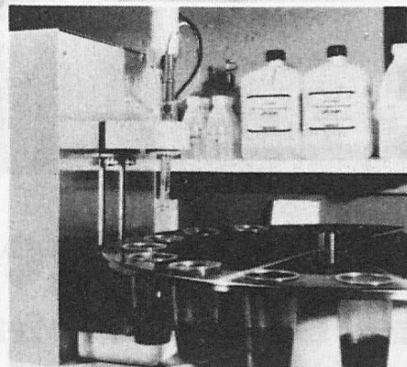
Probenwechsler RT40 mit 16 Probenplätzen für Kleinserien.
