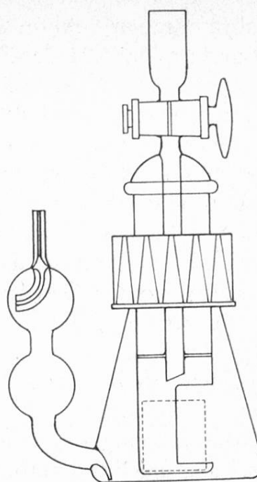
Abb. 2. Neue, verbesserte Apparatur
