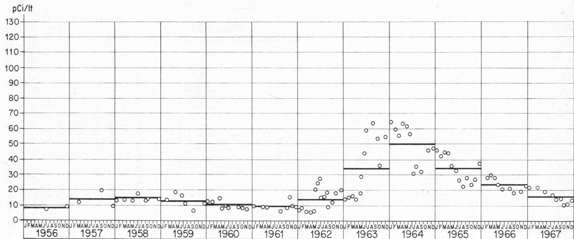
Figure 2 Teneur en strontium-90 du lait en poudre de plaine (canton de Vaud)
