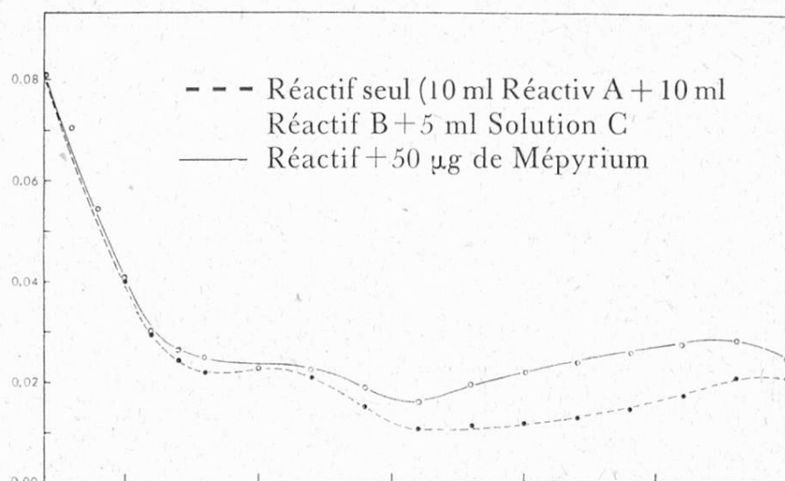
Spectres d'Absorption
