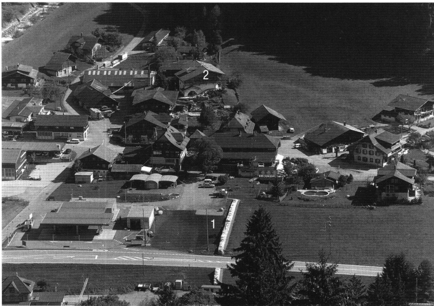
2: Übersicht vom Niesenhang auf Mülmen nach Freilegung und Konservierung der Letzi 1995. Im Vordergrund die neue Umfahrbahnstrasse, welche die Letzi (1) schneidet, im Hintergrund der Weiler Mülmen mit der Burgstelle (2).
