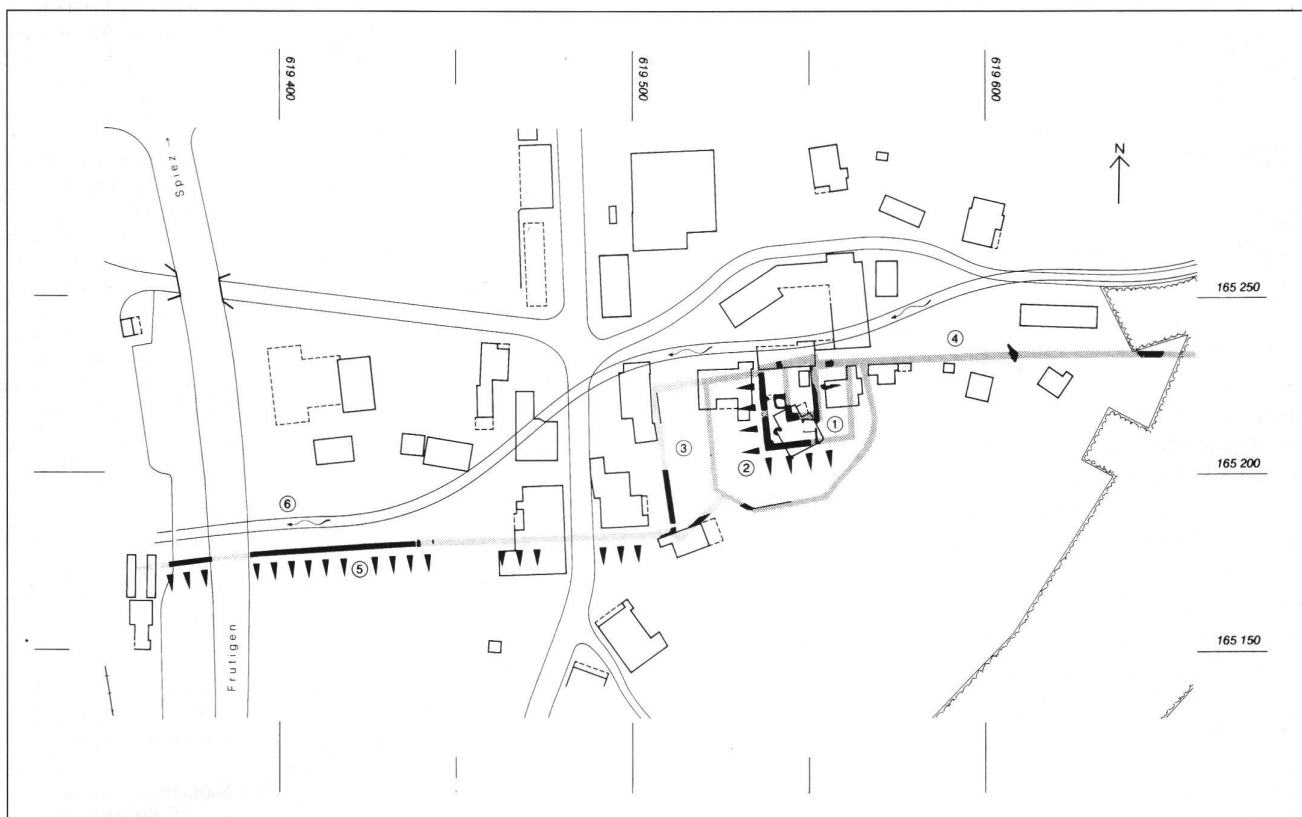
1: Übersichtsplan von Mülönen. M 1:2000. (1) Burg mit zentralem Palas und Ringmauer, (2) Wassergraben mit äusserer Grabenmauer, (3) ummauertes, leicht erhöhtes Plateau (Zwinger, Vorburgbezirk oder «stetli»?), (4) Letzimauer (östlich am Steilhang auslaufend), (5) Letzimauer in der Ebene mit südseitigem Rondenweg, (6) ehemaliger Suldbachlauf (Feindseite).
