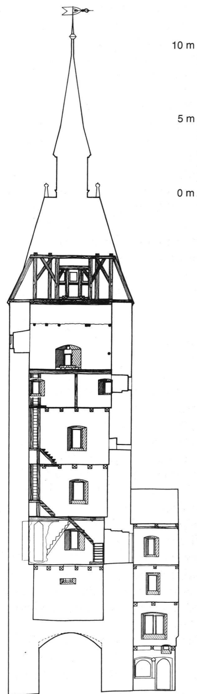
2: Schnitt durch den Spittelturm nach Westen. M. 1:250.
